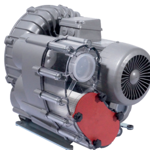
SV 300 inklusive integriertem Ansaugfilter und Vakuumsicherheitsventil
